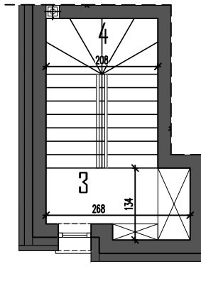
RZUT PIĘTRA
